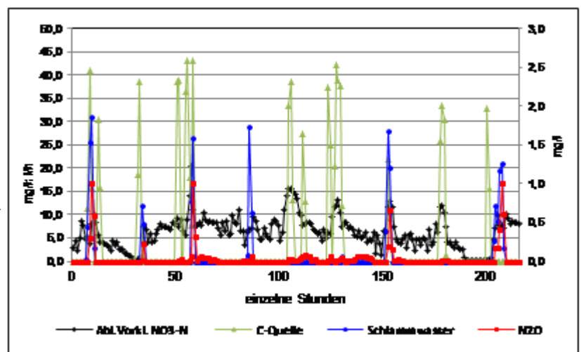
Abb. 3: Grafische Darstellung der Lachgasentwicklung in der Denitrifikationszone.
