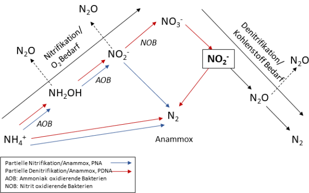
Abb. 1: N 2 O-Formation in Kläranlagen
